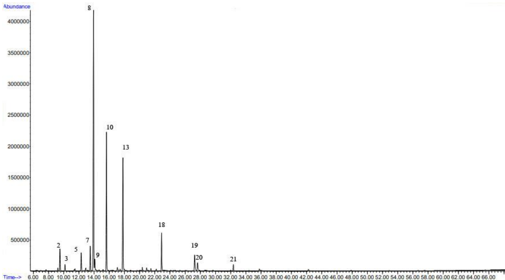
شکل ۱. کروماتوگرام اجزای اسانس مشگک براساس زمان بازداری (اعداد روی هر پیک مطابق با داده های جدول شماره ۱ می باشد)
